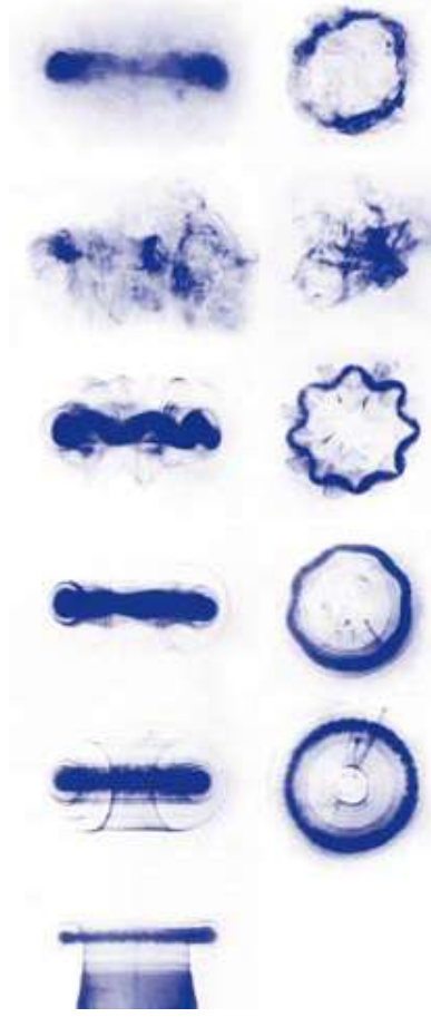
Abb. 6: Wellig werden, Auflösen und neu Formieren eines Ringwirbels. Oben: seitlich und unten entgegengesetzte Laufrichtung gesehen. Bilder vom gleichen Wirbel
