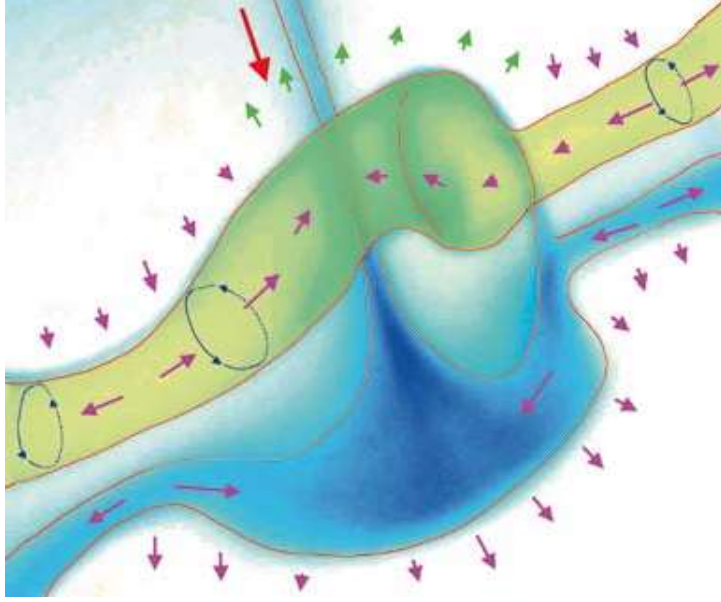
Abb. 11: Strömungen beim Beginn des Abschnürens eines Zwischenwirbels. Aus Stereoaufnahmen geht hervor, dass die Ausbuchtung des Girlandenringwirbels (gelb-grün gefärbt) nach unten in Richtung Schalenboden weist. Bild von schräg oben aufgenommen. Den Versuchsaufbau zeigt Abbildung 13
