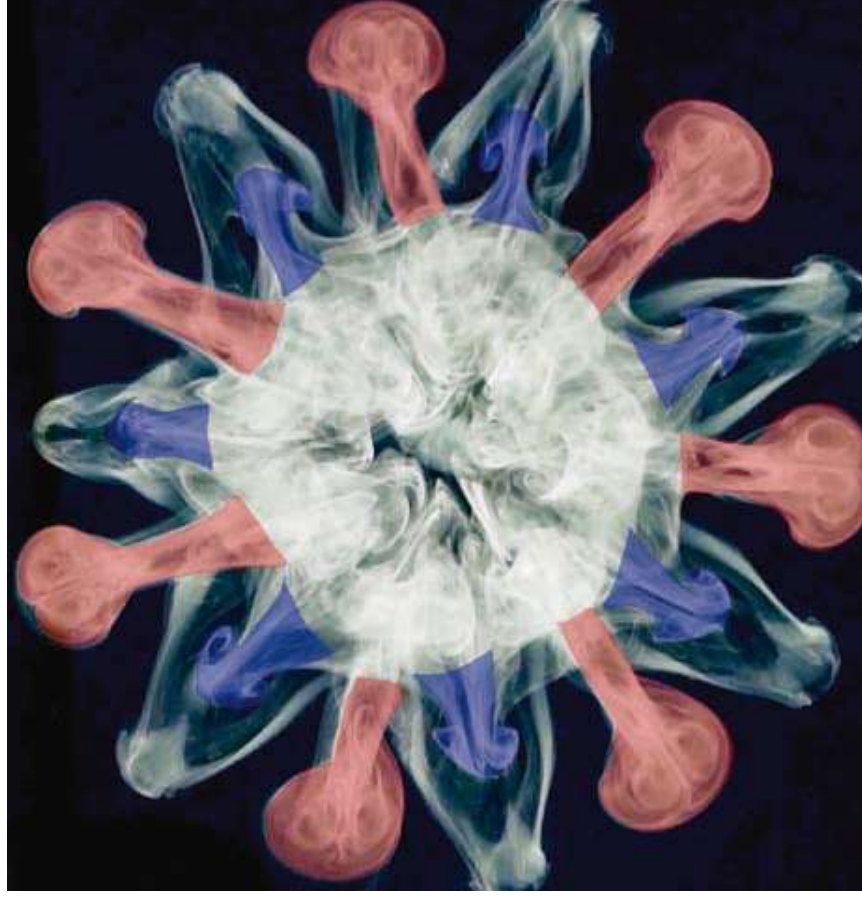
Abb. 3: Ringwirbel, letztes Stadium, mit auf Foto eingefärbten Wirbeln
