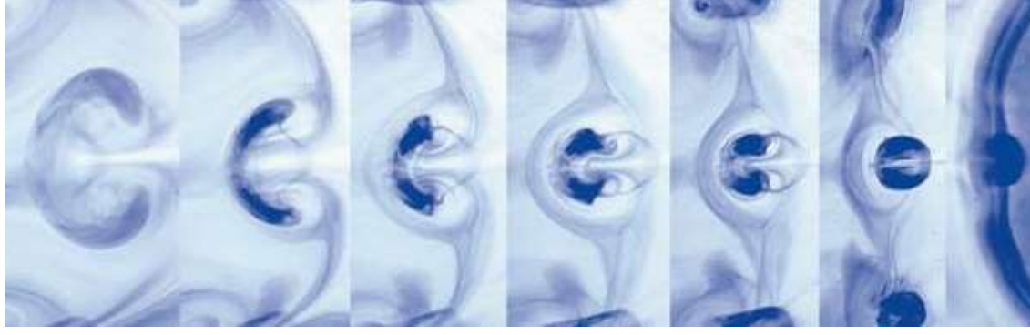
Abb. 20: Entwicklung eines Zwischenwirbels durch Abschnüren aus einem Teil des G-Ringwirbels
