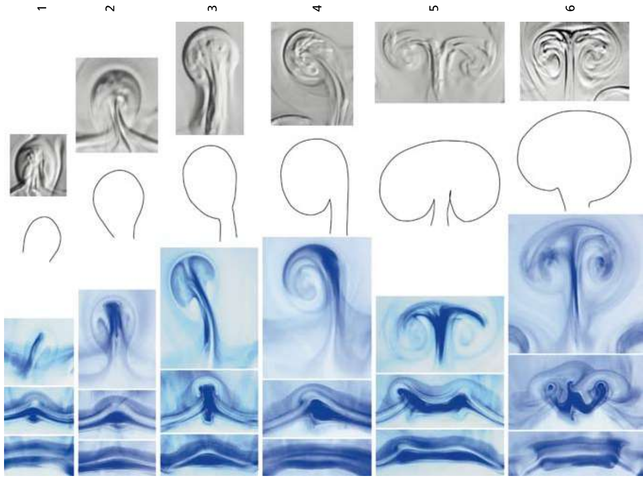
Abb.14: Erscheinungsformen der Primärwirbel
