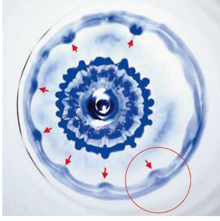
Abb. 7: Girlandenringwirbel. Pfeile markieren zurückbleibende Ausbuchtungen nach unten
